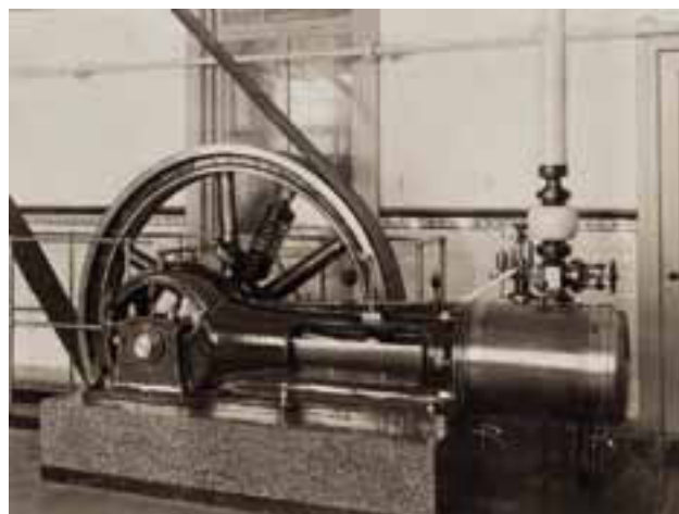
De Stork éencilinder A46 stoommachine welke in 1915 werd geplaatst
